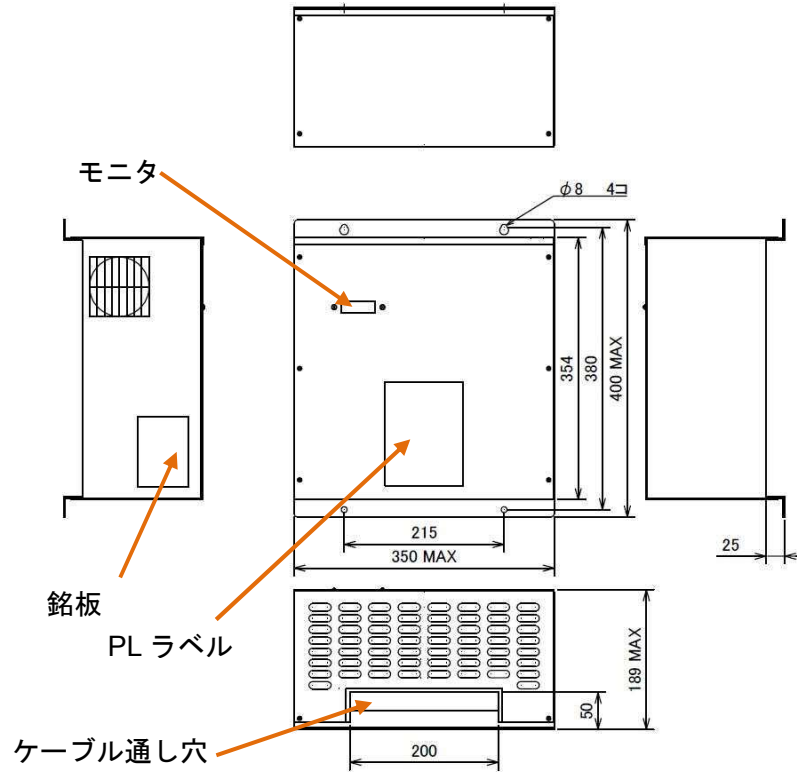
図 2-8 モータドライバの寸法
