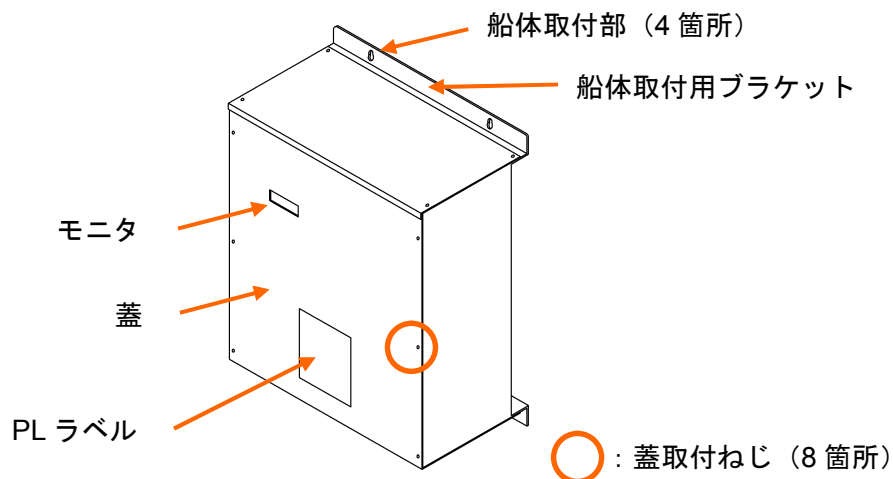
図 2-7 モータドライバ本体の外観形状
