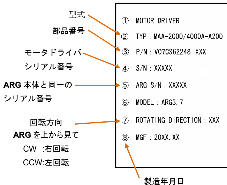
図 2-9 モータドライバの銘板
