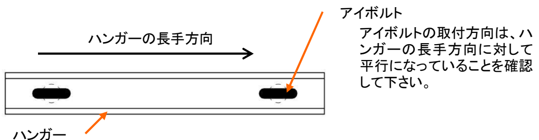
図 4-3 ハンガーのアイボルト取付方向
