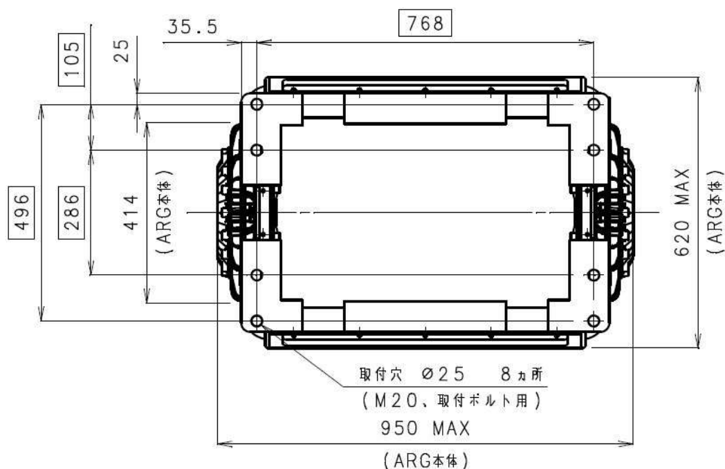
図 4-1.1 ARG 本体の取付穴寸法
